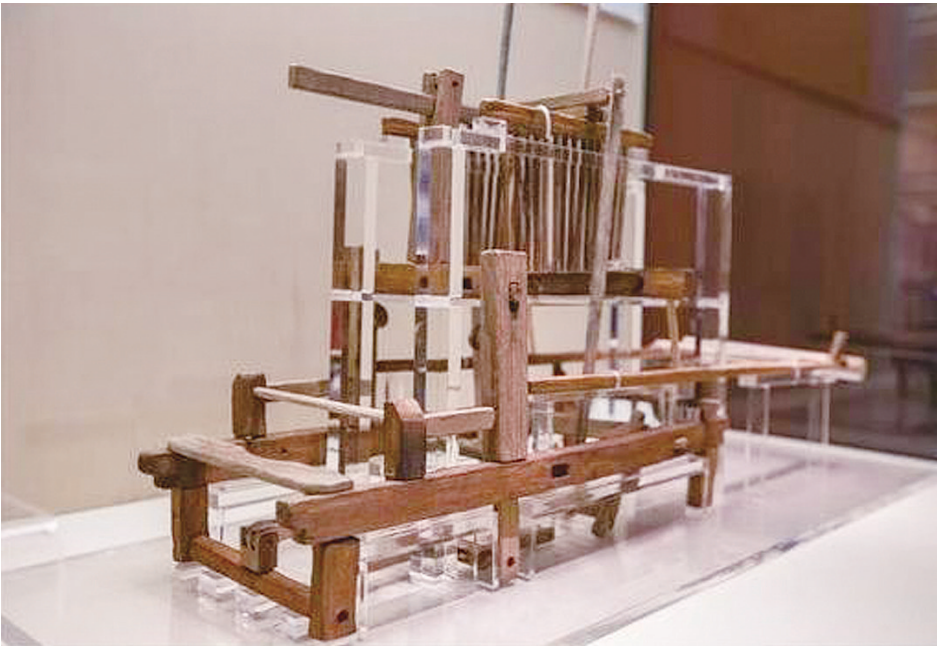
老官山汉墓蜀锦提花机
